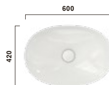
L4706E#XW Aufsatzwaschtisch TL rund 600mm, ohne Hahnloch, ohne Überlauf, mit Schaftventil TL vessel round 600mm, without tap hole, without overflow, incl. stem valve
