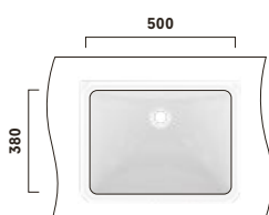
LW1535Y Unterbauwaschtisch WU, eckig 500mm, ohne Hahnloch, mit Überlauf Undercounter basin WU square 500mm, without tap hole, with overflow
