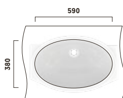
LW1506JUYW/F#W Unterbauwaschtisch WU, rund 600mm, ohne Hahnloch, mit Überlauf Undercounter basin WU round 600mm, without tap hole, with overflow
